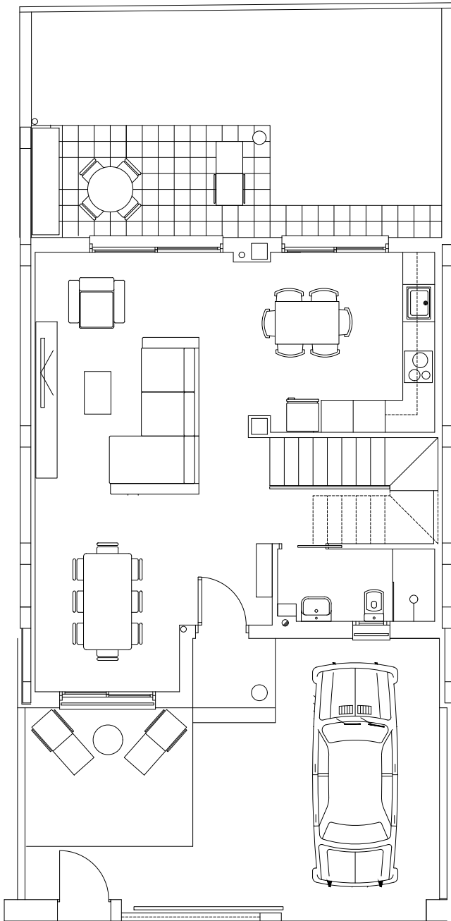
PLANTA BAJA
