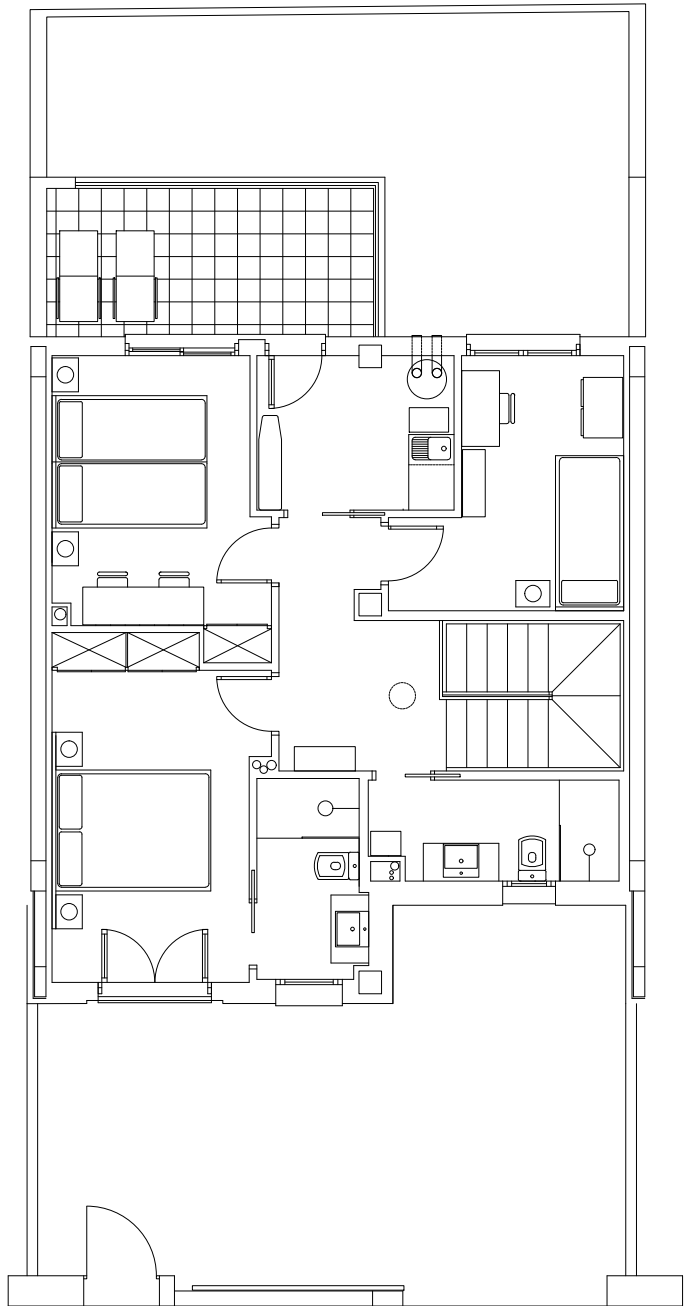
PLANTA PRIMERA
